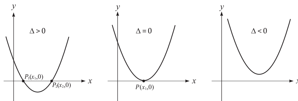
Figura 12: Discriminante
