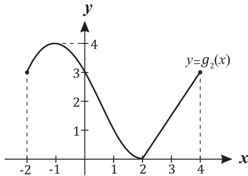
Figura 9: g_2
