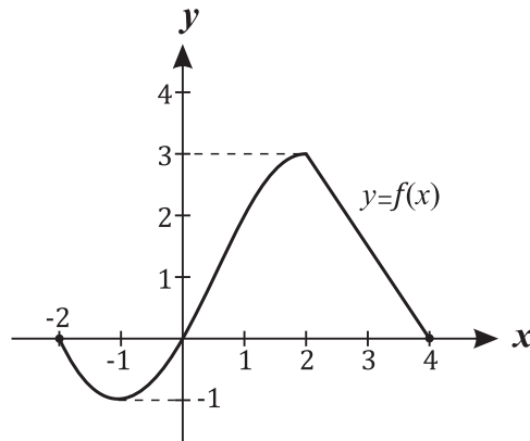
Figura 7: f
