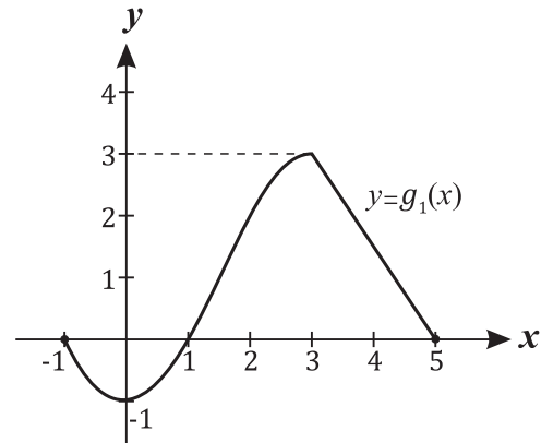
Figura 8: g_1
