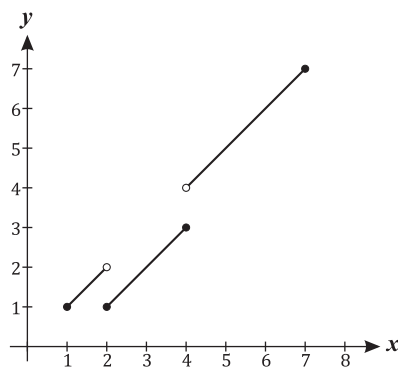
Figura 1: y = f(x)
